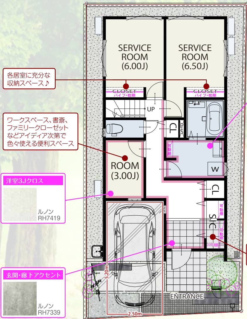
1 FLOOR / 61.11㎡ (車庫面積10.18㎡含む)
