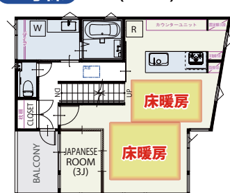
2号棟 LDK(19.6J)
