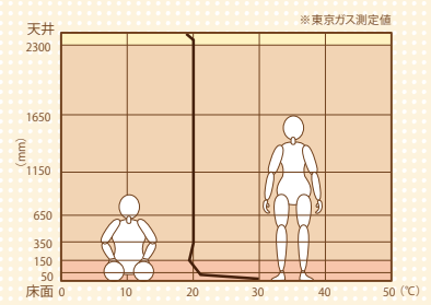
床暖房の垂直温度分布
