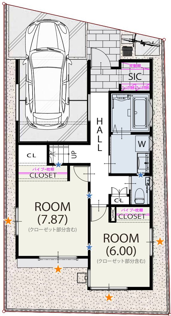
1 FLOOR / 57.34㎡ (車庫面積14.49㎡含む)
