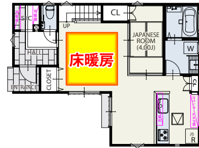
2号棟 LDK:17.25J
